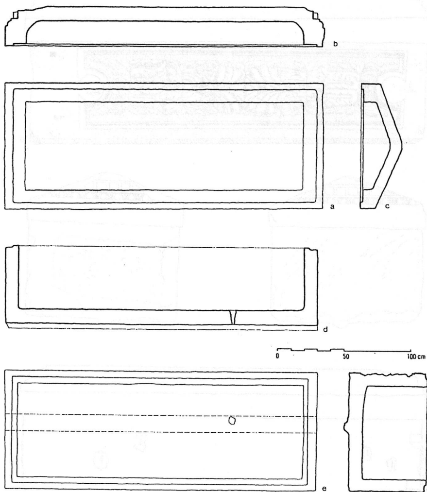
Sl. 2. Galovac-Crkvina: a- uzdužni presjek poklopca sarkofaga, b- pogled na sanduk odozgora, c- poprečni presjek poklopca, d- uzdužni presjek sanduka, e- pogled na dno sanduka, f- bočni presjek sanduka. – Fig. 2. Galovac-Crkvina: a- longitudinal section of the sarcophagus lid, b- view of the sarcophagus from above, c- vertical section of the lid, d- horizontal section of the trunk, e- bottom view of the trunk, f- side-section of the trunk.
