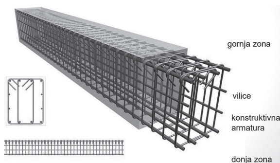
Slika 2. Krutost kaveza
