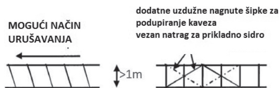
Slika 3. Oblik armature
