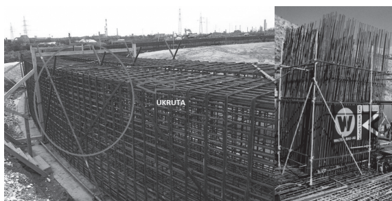
Slika 4. Osiguranje konstrukcije
