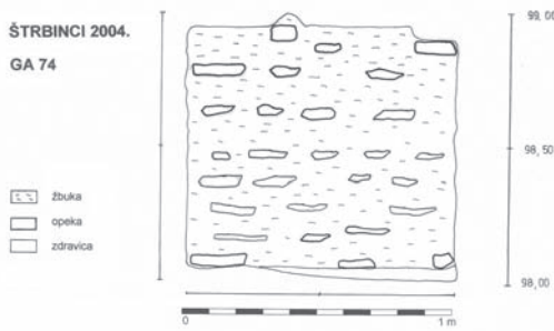
Sl. 4. GA 74 - zapadni zid izvana
