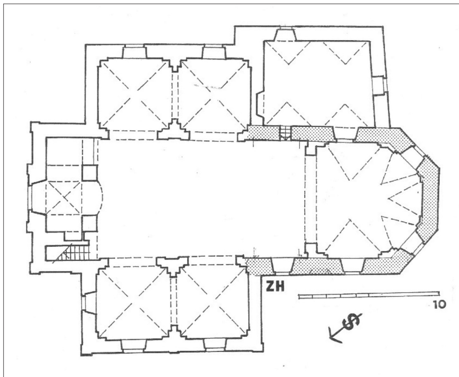
Sl. 4. Slunj, župna crkva Presvetog Trojstva, tlocrt: rasterom označen srednjovjekovni dio crkve (crtao: Z. Horvat)
