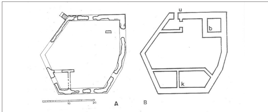
Sl. 18. Slunj, utvrda (burg), tlocrt: A) Tlocrt ruševina burga 14. - 15. st. - snimka prije 1991. godine; B) Pokušaj rekonstrukcije tlocrta burga, s naznačenom kapelom K (crtao: Z. Horvat)
