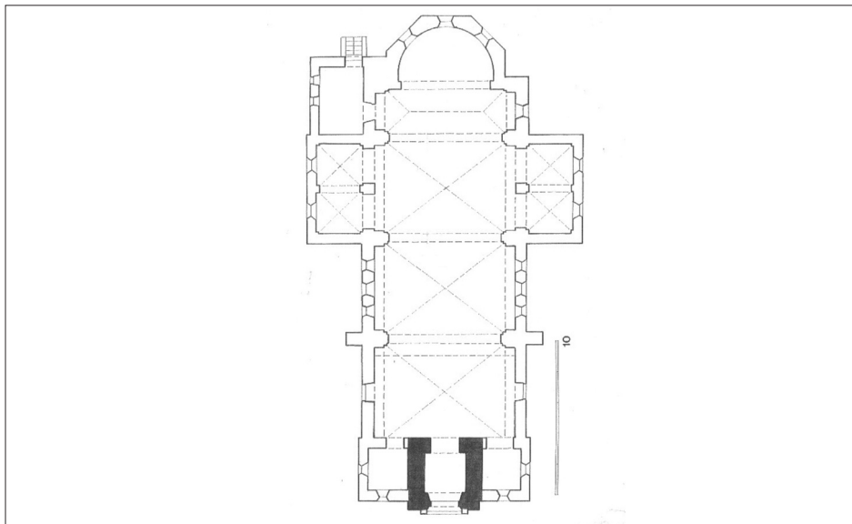
Sl. 21. Cvitovići kraj Slunja, župna crkva sv. Nikole, tlocrt: crkva građena početkom 20. st., a zvonik je još ostatak srednjovjekovne građevine (crtao: Z. Horvat prema podlozi iz Konzervatorskog zavoda Karlovac)
