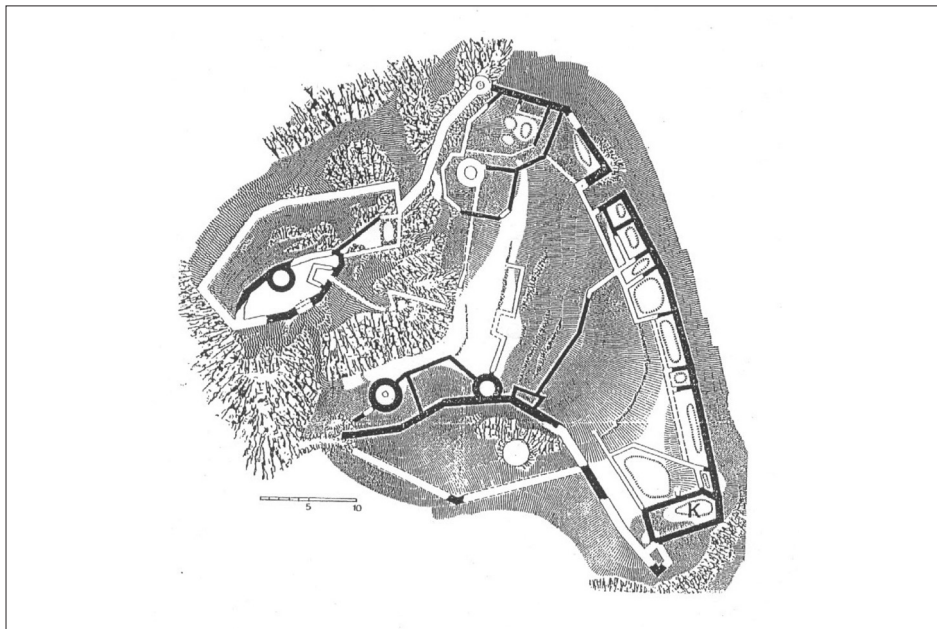
Sl. 20. Komčić-Karlovića Dvori, burg, tlocrt: K – vjerojatna kapela (crtali: F. Ilakovac i V. Henneberg, 1934. godine, original u Ministarstvu kulture, UZKB, Planoteka)
