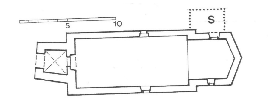
Sl. 19. Brinje, Humac, kapela sv. Vida, tlocrt (crtao: Z. Horvat)
