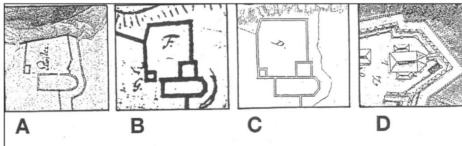
Sl. 16. Tlocrti slunjskog franjevačkog samostana s crkvom tijekom vremena: A) Stier, 1660.; B) Marsigli, oko 1700.; C) Weiss, 1730.; D) Projekt uređenja barokne (?) utvrde oko Slunja potkraj 18. st. 29
