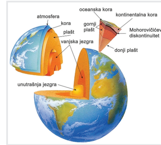
... građa unutrašnjosti Zemlje
