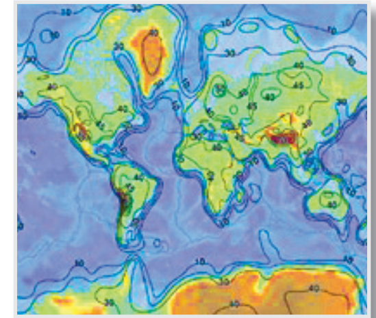
... karta dubina Mohorovičićevog diskontinuiteta
