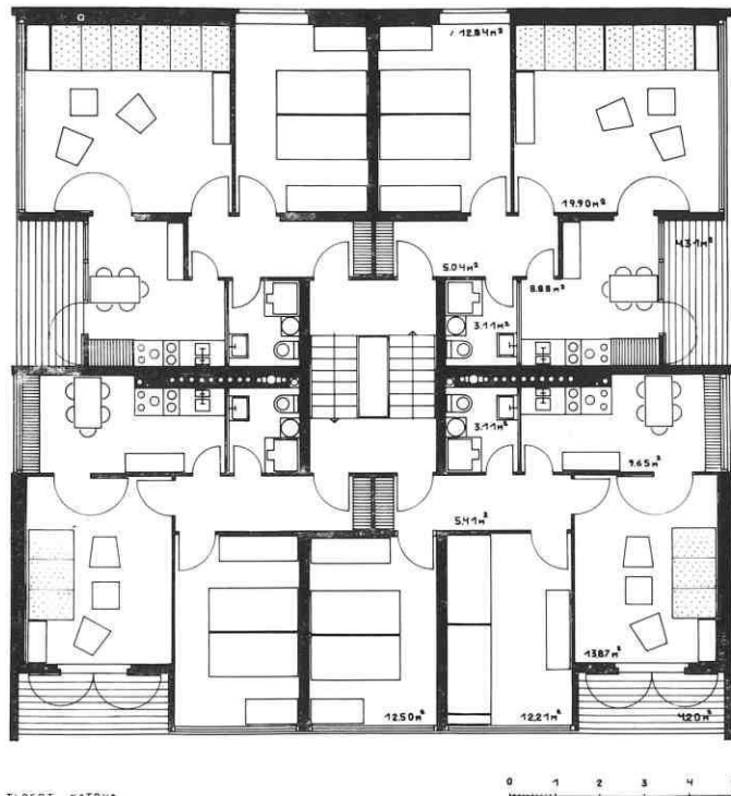
TLOCRT KATOVA
