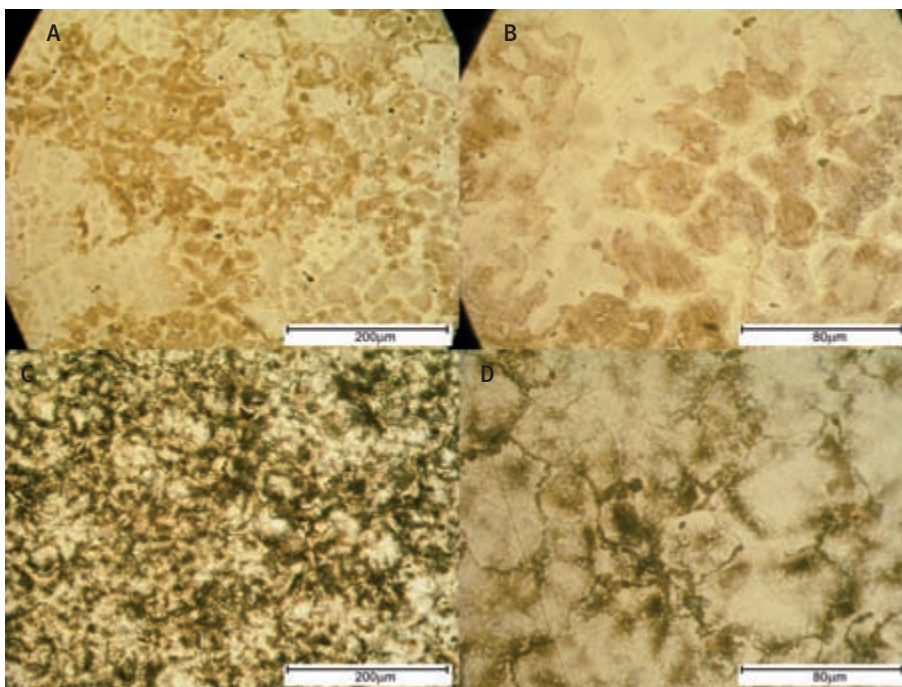
Slika 2. Mikrografske snimke pod različitim povećanjima odljevka Dentora S (A) i (B), i odljevka Midora S (C) i (D).
