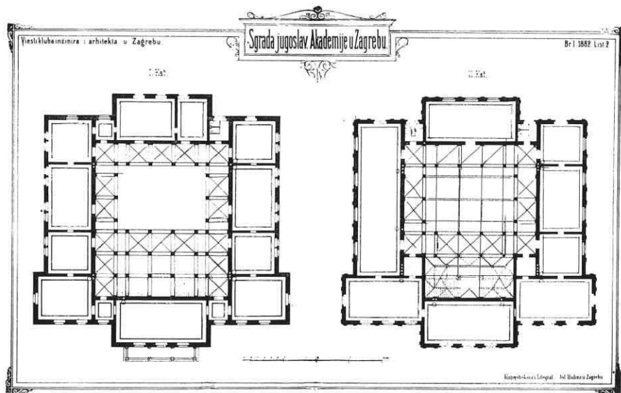
Tlocrt I. i II. kata palače Akademije u Zagrebu, izvedbeni nacrti
