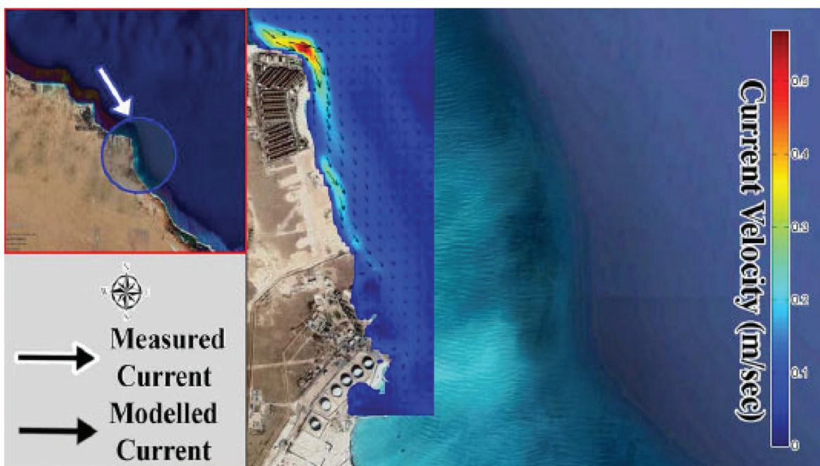
Figure 17 Calibration status for measuring currents in the study area Slika 17. Kalibracija za mjerenje struja u području istraživanja
