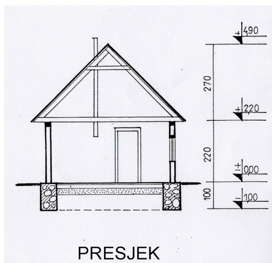
2. Arhitektonski nacrt – presjek kroz zgradu, mr. T. Arsenić, 1999.
