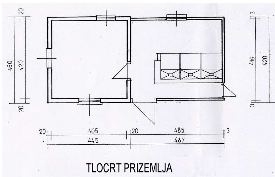
3. Arhitektonski nacrt s vidljivim dvoprostornim rasporedom unutrašnjosti i pozicijom mlinskog postrojenja. Snimila: mr. T. Arsenić, 1999.
