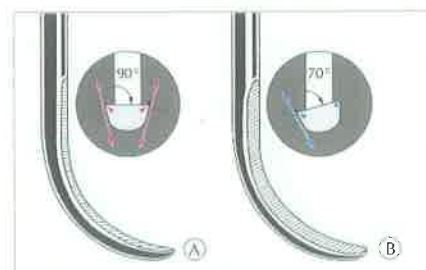
Slika 6. Razlika između univerzalnih i Gracey kireta. (2)
