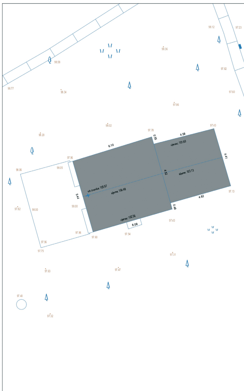
Slika 3. Tlocrt crkve, geodetski snimak, izradio dipl. ing. geod. Toni Tadin
