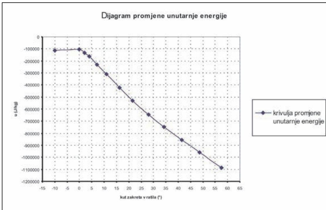
Slika 5. Promjena vrijednosti unutarnje energije u funkciji kuta zakretanja \varphi Figure 5. Internal energy value change in function of crank angle \varphi
