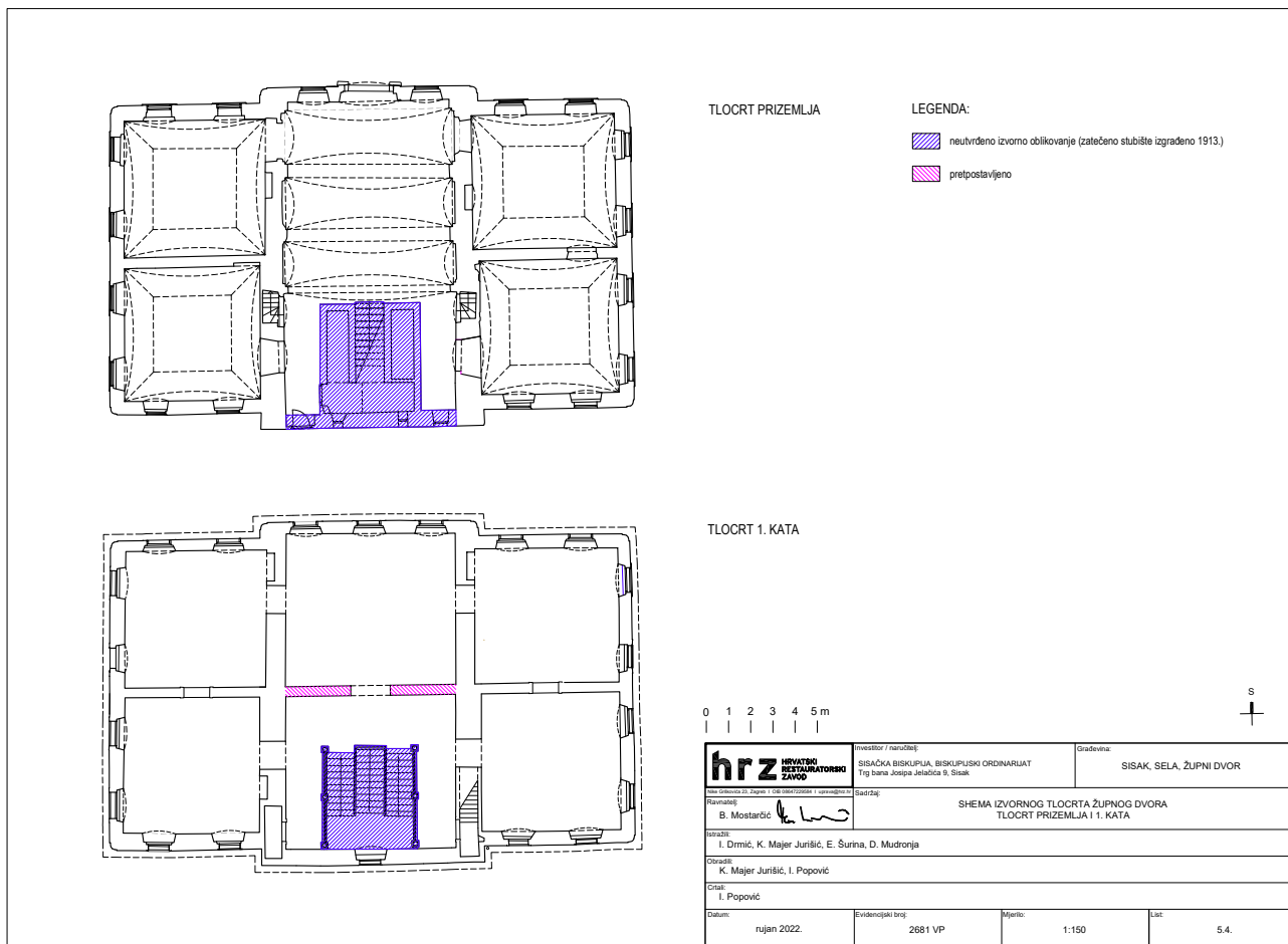
16 Župni dvor u Selima, pretpostavljeni izvorni tlocrt prizemlja i kata (crtala: I. Popović, (dokumentacija HRZ, 2022.)
