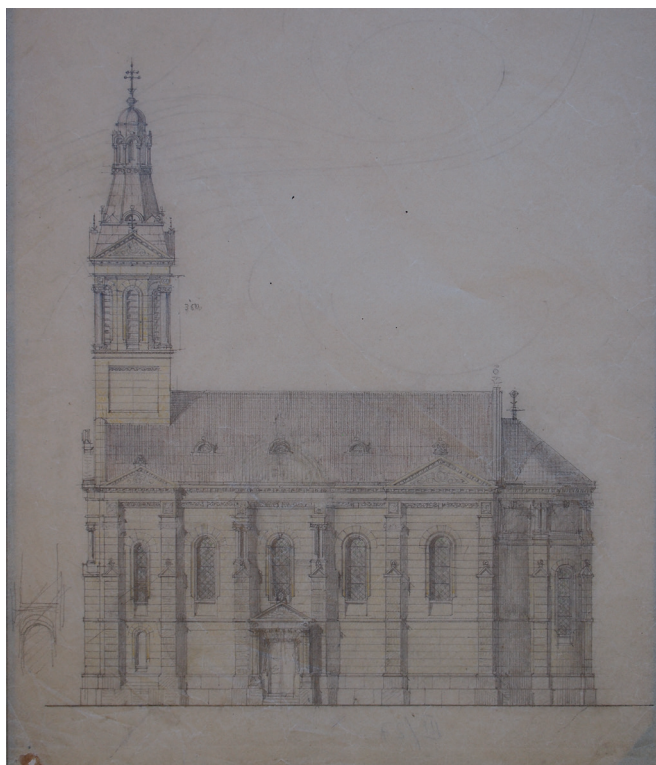
12. Herman Bollé, Projekt za restauriranje bočne fasade parohijske crkve Preobraženja Gospodnjega u Zagrebu, 1913; NAZ (Nadbiskupijski arhiv Zagreb), ZNDM (Zbirka nacrti dijecezanskog muzeja), sign III-27.
