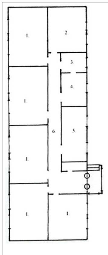
Slika 5. Paviljonska školska zgrada s šest učionica i ostalim potrebnim prostorom 1961. godine
