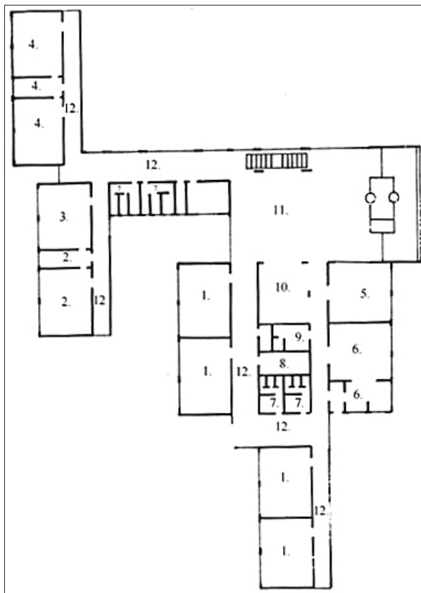
Slika 6. Suvremena školska zgrada sa specijaliziranim učionicama i ostalim pratećim prostorom, prizemlje 1978. godine
