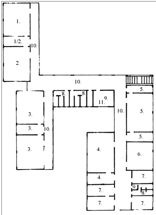
Slika 7. Suvremena školska zgrada sa specijaliziranim učionicama i ostalim pratećim prostorom, kat 1, 1978. godine
