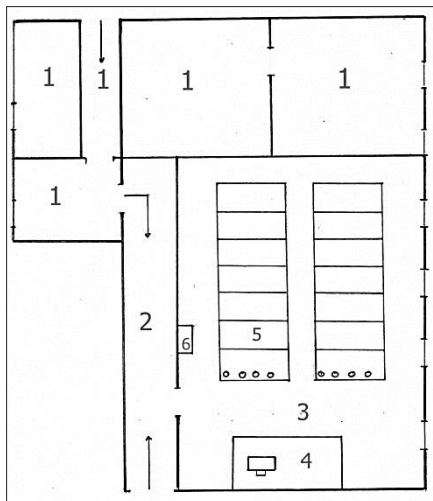
Slika 1. Jednorazredna školska zgrada s učiteljskim stanom 1890. godine
