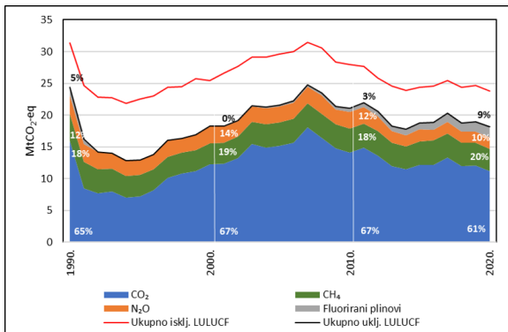
(c) Doprinosi stopi promjene u odnosu na baznu godinu, HR
