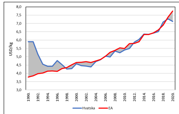
(b) Produktivnost emisije CO_2^{**}
