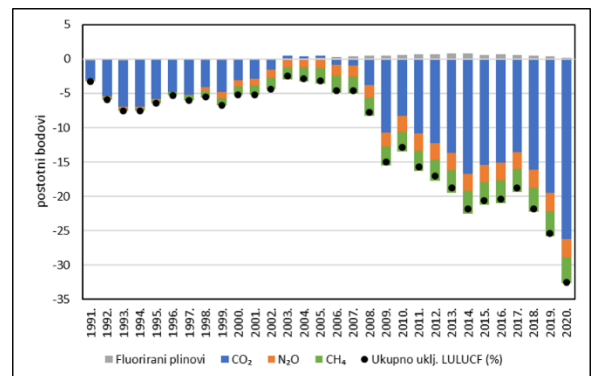
(f) Doprinosi godišnjoj stopi promjene, EA
