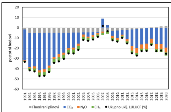
(e) Doprinosi godišnjoj stopi promjene, HR
