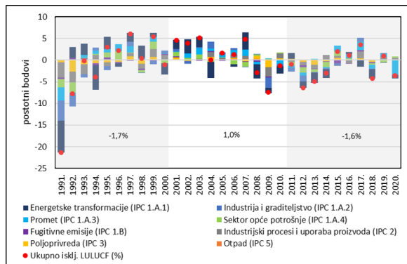
(e) Doprinosi godišnjoj stopi promjene, HR (f) Doprinosi godišnjoj stopi promjene, EA
