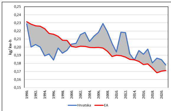
(a) Intenzitet emisije CO_2^*
