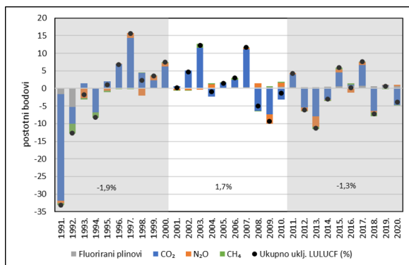
(e) Doprinosi godišnjoj stopi promjene, HR
