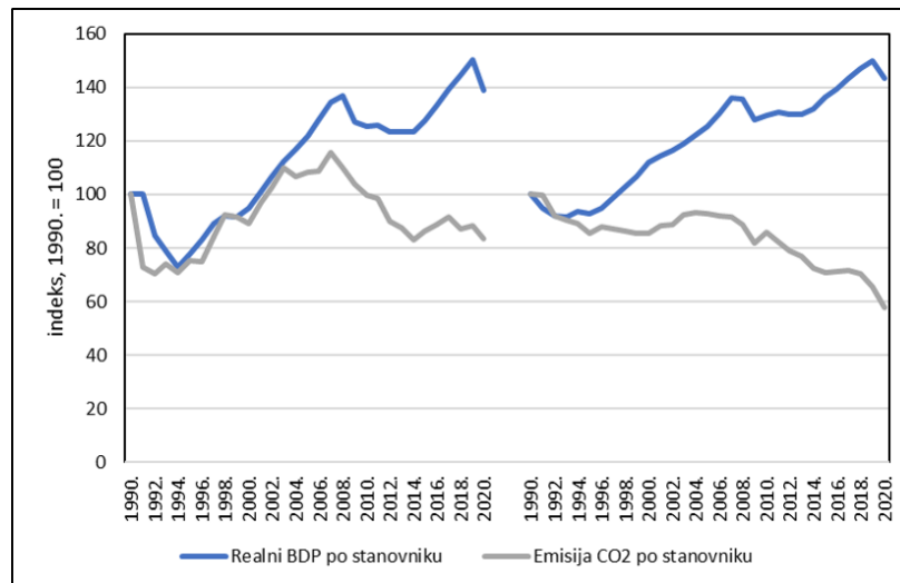
Slika 2. Kretanja emisije CO 2 po stanovniku i realnog BDP-a po stanovniku u Hrvatskoj (lijevo) i europodručju (desno)
