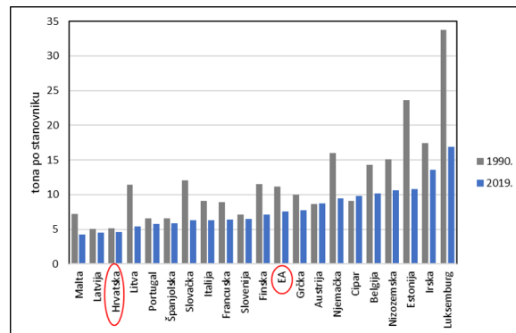
(c) Emisije po stanovniku po zemljama članicama EA u 1990. i 2019.**
