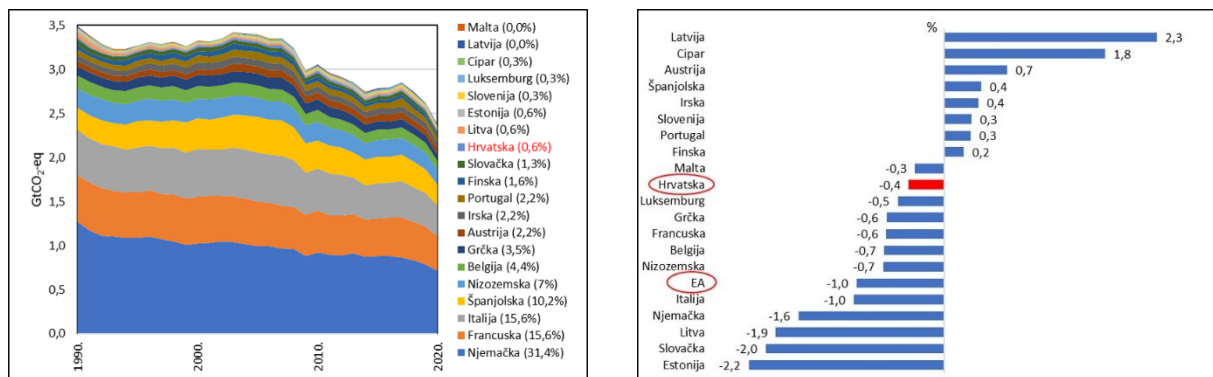
(a) Kretanja ukupnih emisija EA i prosječni godišnji doprinosi zemalja ukupnim emisijama (u zagradi u %)
