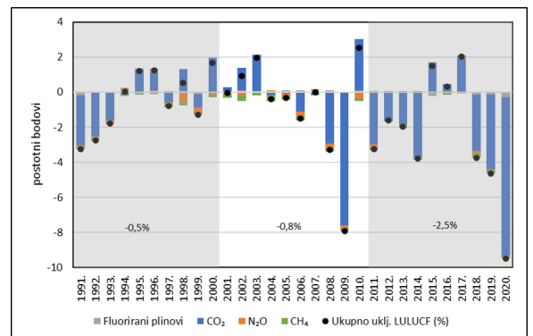
(f) Doprinosi godišnjoj stopi promjene, EA
