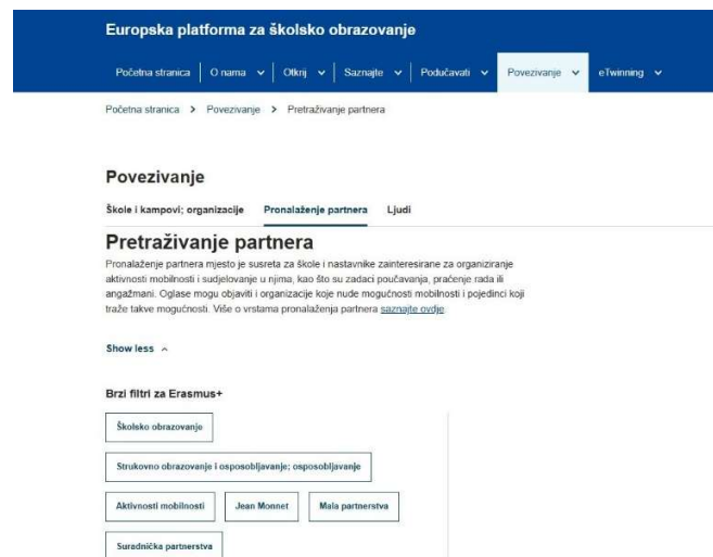
Slika 10 - Pretraživanje partnera
