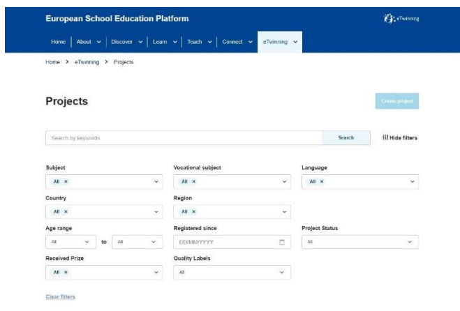
Slika 11 - Pretraživanje projekata
