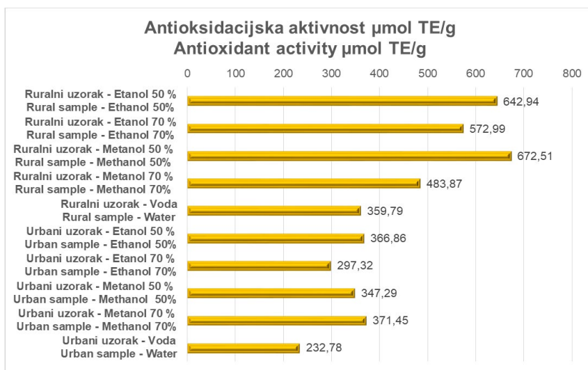
Grafikon 2. Rezultati DPPH metode za uzorke izraženi primjenom standarda Trolox-a kao ekvivalenta ( \mu\text{mol TE/g} ). Graph 2. Results of DPPH method for samples expressed using Trolox standards as equivalents ( \mu\text{mol TE/g} ).
