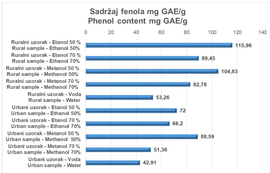
Grafikon 1. Srednje vrijednosti ukupnih fenola u ovisnosti od primijenjenog otapala i nadmorske visine. Graph 1. Mean values of total phenols depending on the applied solvent and altitude.
