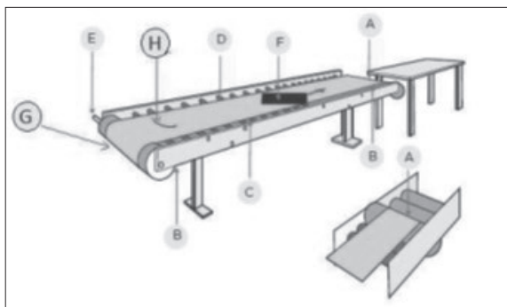
Slika 3. Opasnosti pri radu s trakastim transporterima
