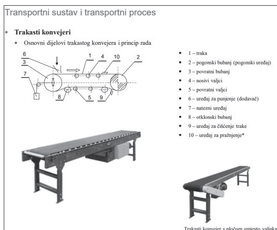
Slika 2. Trakasti transporter
