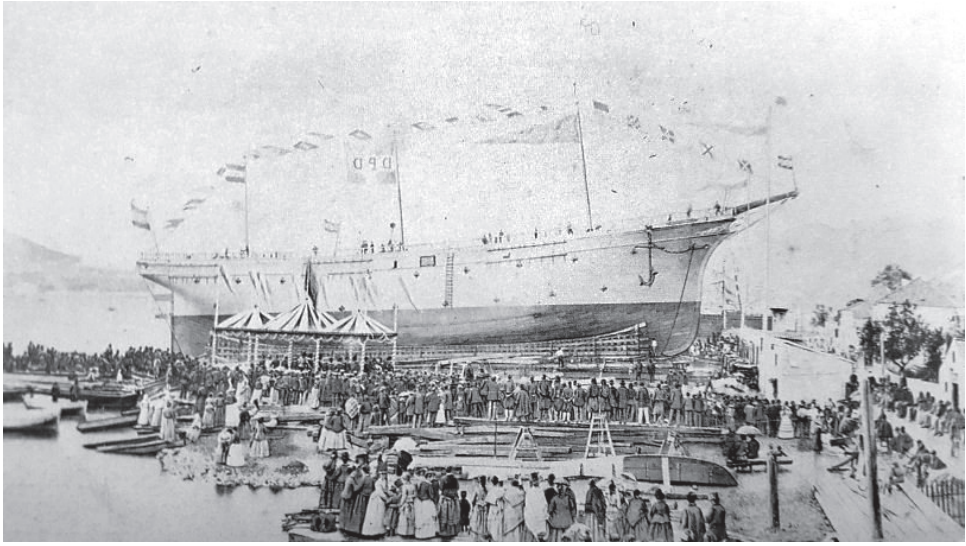
Slika 2. Porinuće nave Dvanaesti Dubrovački. Izvor: Album fotografico-illustrativo del viaggio di S. M. L'imperatore e re Francesco Giuseppe I. in Dalmazia nel 1875 . Zara: 84.
