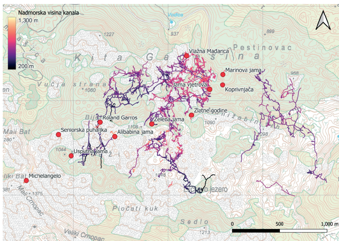
Tlocrtni prikaz poligonskih vlakova JSC-a i Munižabe obojenih prema nadmorskoj visini i objekata u kojima je zabilježeno snažno strujanje zraka Priredio: Dino Grozić
