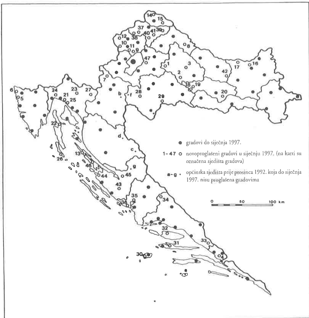
Sl. 2. Sjedišta gradskih područja u Republici Hrvatskoj.
