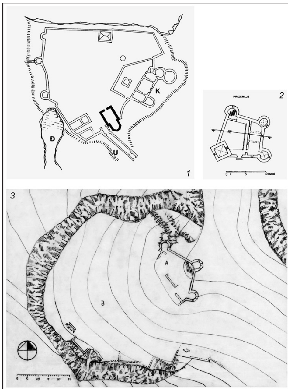
Usporedni prikaz tlocrta: 1. Ogulin, 2. Dubovac, 3. Grižane (Regan K. 2005; Horvat 1997a, 147; Kruhek M. 1995, 104)
