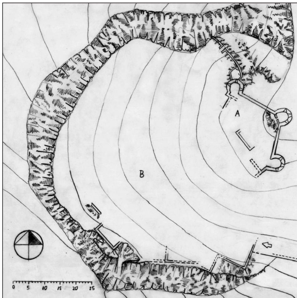
Skica tlocrta ostataka grižanskog plemićkog grada: A – gradska jezgra, B – utvrđeno predgrađe (Regan K. 2005.)
