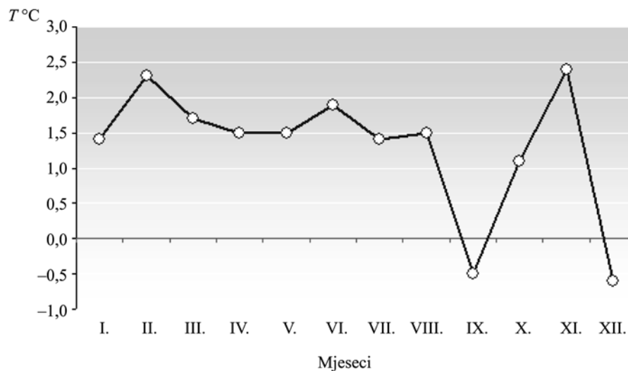
Slika 4. Usporedba srednjih mjesečnih temperaturnih krivulja prvog (1979.–1988.) i trećeg (1999.–2007.) desetljeća
