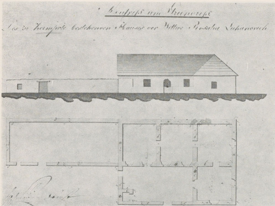
Nacrt i tlocrt kuće i staja koju je krajiška uprava podigla udovici Rozaliji Luka- nošić u Krmpotama. Izradio graditelj Malinarić (Arhiv Hrvatske — zbirka: Planovi — mape, br. 142)
