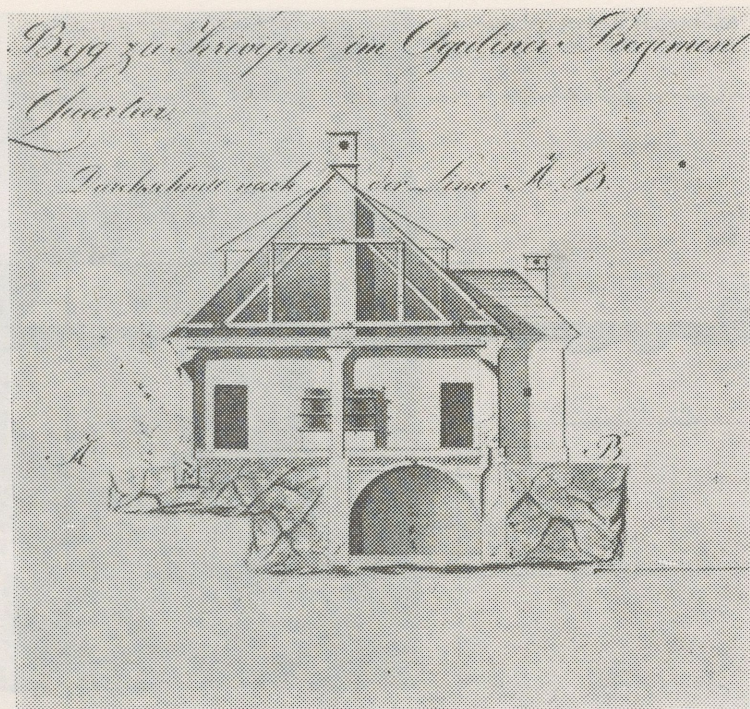
Presjek oficirskog stana krmpotske satnije u Krivom Putu. Crtež majora Božičevića iz 1822. godine. (Arhiv Hrvatske — zbirka: Mape — planovi, br. 210)
