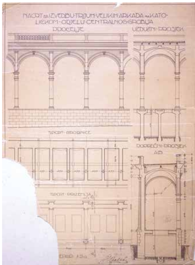
9. Herman Bollé, Projekt za velike arkade katoličkog odjela (dio smješten između evangeličkih i pravoslavnih arkada) na Mirogoju, 1912. (NAZ-ZNDM, sign. III-42, Mirogoj)
