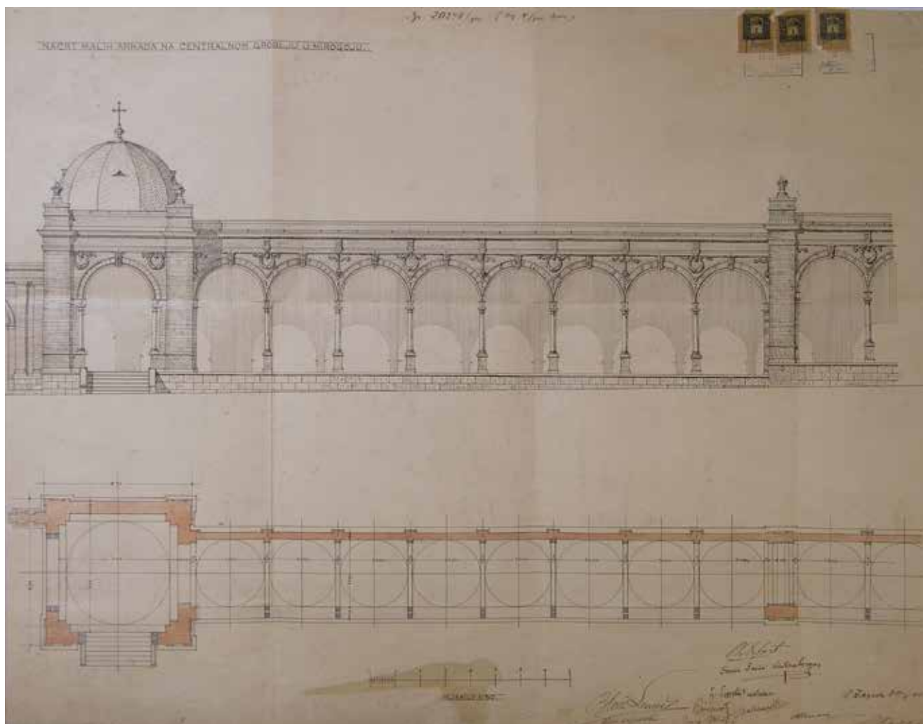
13. Herman Bollé, Izvedbeni projekt za male arkade, 1905. (HR-DAZG-4, Gradsko poglavarstvo Zagreb, kut. 1878.)
