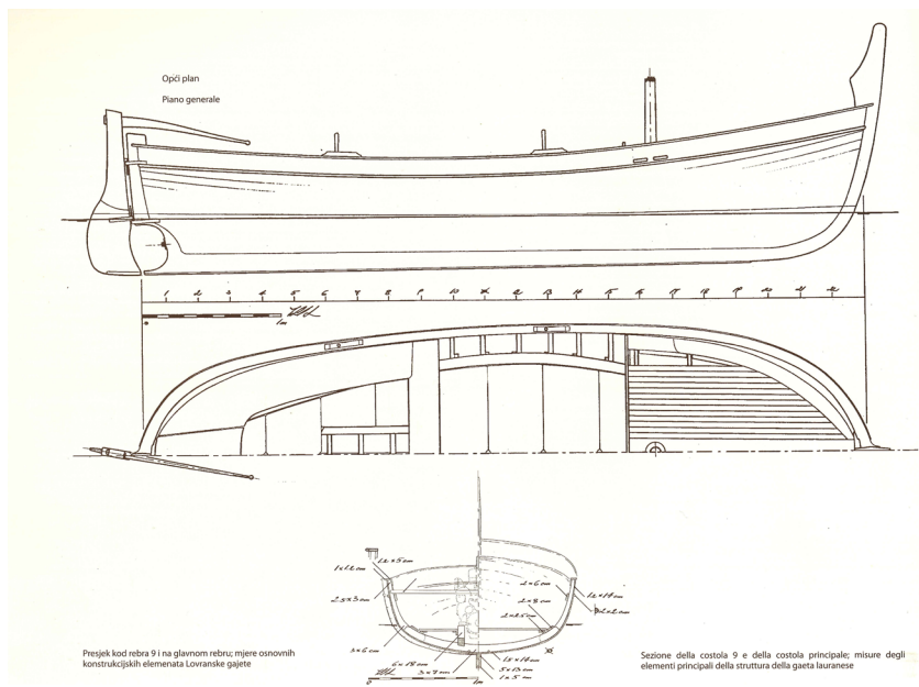
Slika 3. Kuća lovranskoga guca - nacrti (2)
