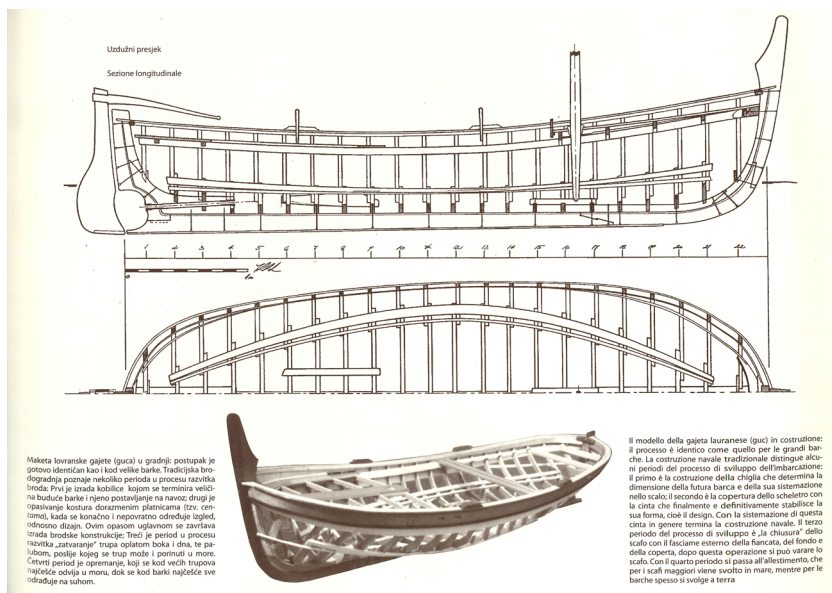
Slika 2. Kuća lovranskoga guca - nacrti (1)
