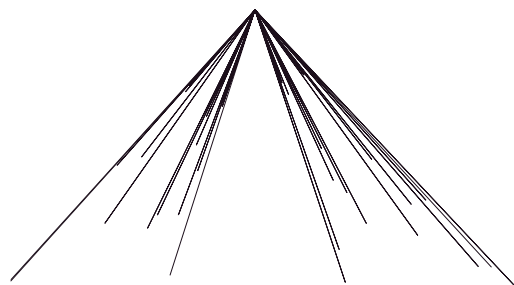
FIGURE 2.2. A Lelek fan
