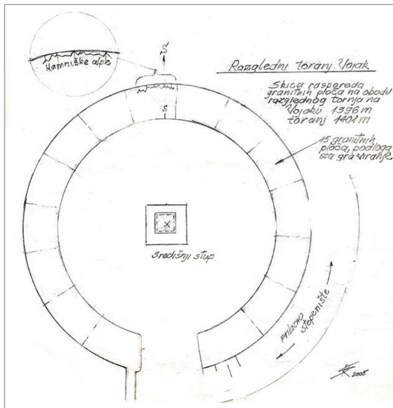
Slika 7. Skica rasporeda granitnih ploča za graviranje točaka na horizontu na obodu razgledne kule na Vojaku. (Knjiga 3: 14. 10. 2005.)
