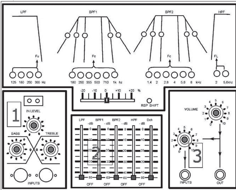
shema SUVAG uređaja
