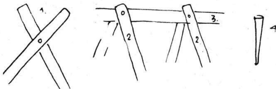
7. slika — Povećani pojedini dijelovi krova kao i drenov klin 1. škare, 2. konji, 3. slime (sljeme), 4. drijenov klin.
