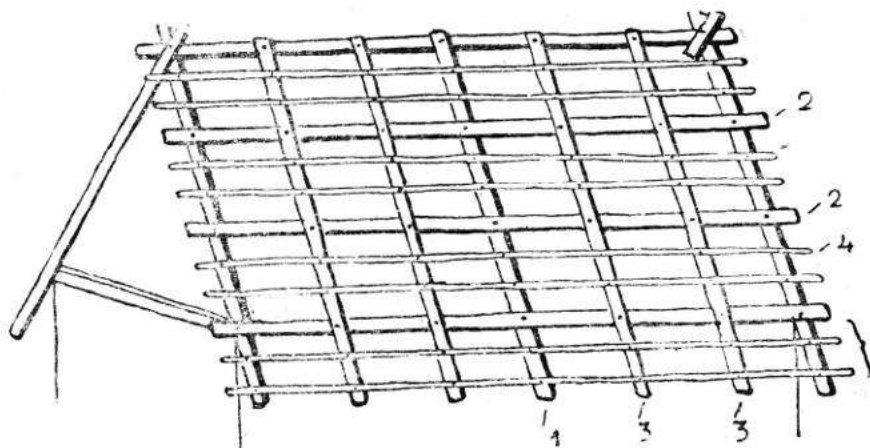
6. slika — Dovršena konstrukcija krova 1. konj, 2. porebrnice, 3. limezi, 4. rebra ili litve, 5. grondav ili grandal
