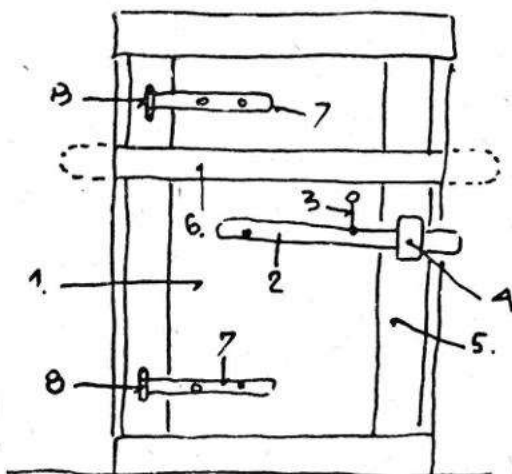
3. slika — Vrata gledana iznutra
