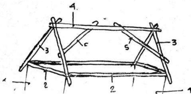
5. slika — Početni sastav krova 1. zidovi, 2. pomernici, 3. škare, 4. slime, 5. lejštre.
