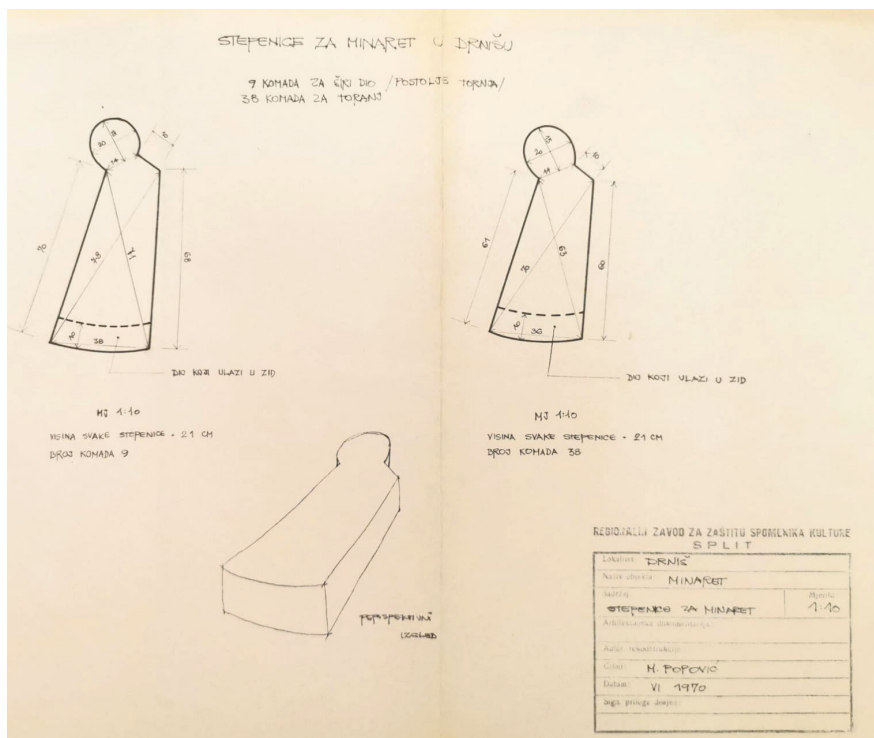
Sl. 6. Projekt rekonstrukcije stubišta za minaret u Drnišu, lipanj 1970. (MK – UZKB – KOS, autor Mladen Popović, Stubište za minaret u Drnišu, lipanj 1970.)
