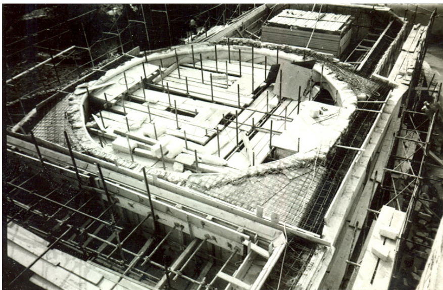
Sl. 9. Radovi na kupoli sv. Ante u Drnišu (MK – UZKB – KOS, Inv. br. 95722, Armatura oko podnožja kupole, autor Goran Nikšić, kolovoz 1989.)
