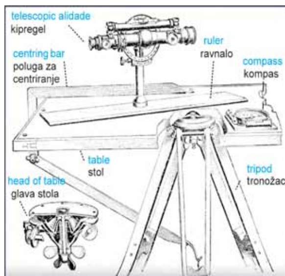
Fig. 12. A plane table with alidade Wild from 1927 Slika 12. Geodetski topografski stol s kipregelom Wild iz 1927. godine
