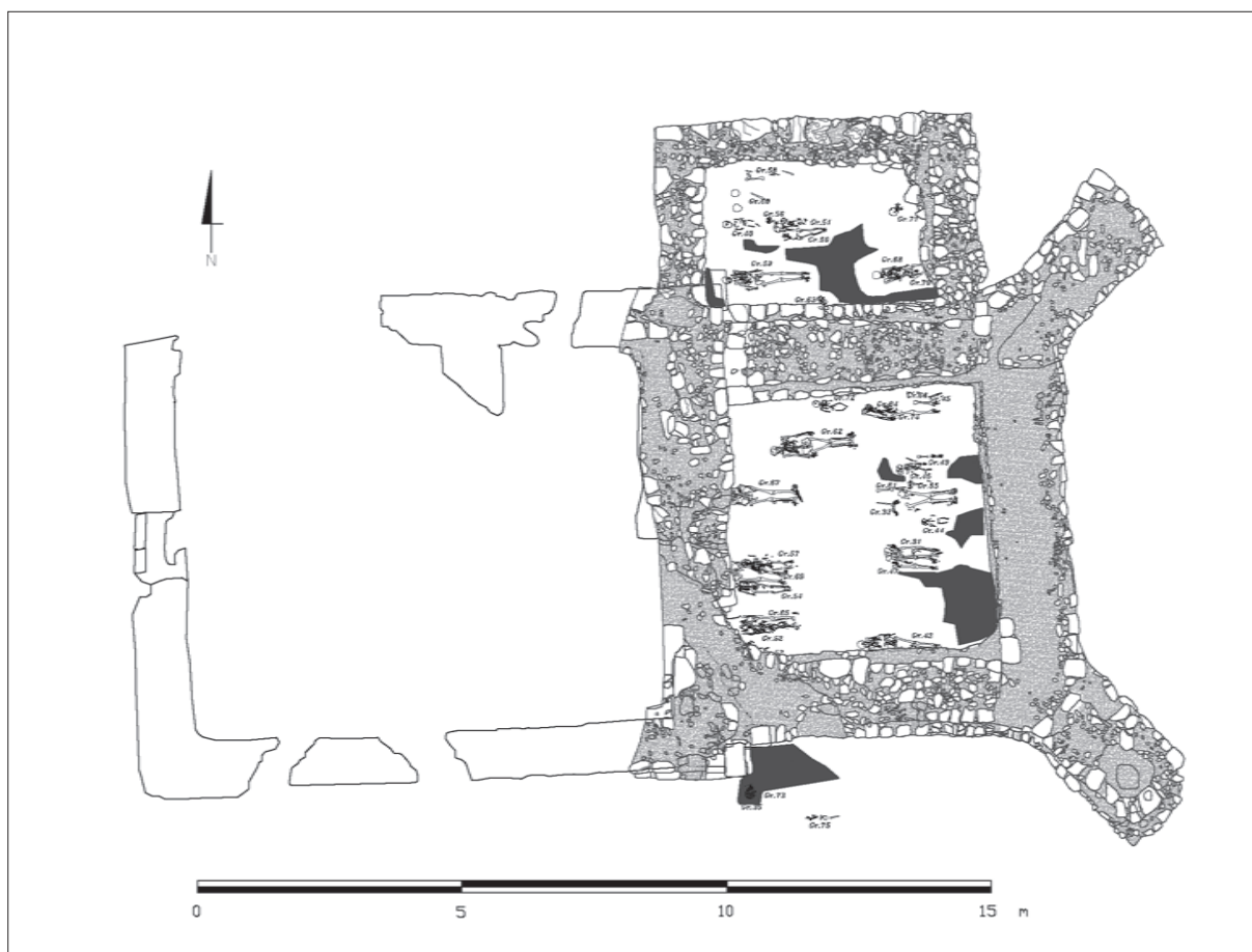
Sl. 1. Ivanec – Stari grad, tlocrt crkve Sv. Ivana s nalazima kampanje 2007. (izradile: Nela Kovačević i Andreja Kudelić)
