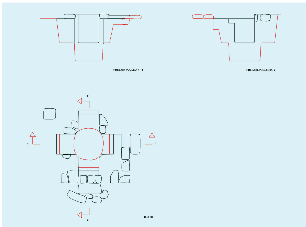
Sl. 6. Tloris krsnog zdenca.
