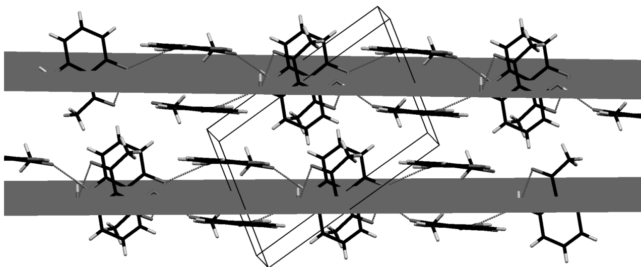
Slika 5 – Dvodimenzionalna mreža vodikovih veza: prikaz ravnina u kristalnoj strukturi dihidroxiacetofenona 16 načinjen programom Mercury. 13 Spoj se primjenjuje u spektrometriji masa kao matrica za vezivanje analizirane supstance. Nije poznato o čemu ovise dobra svojstva matrice. Pretpostavlja se da matrica s hidrofilnim graničnim slojem "pogoduje" interakcijama s hidrofilnim površinama analizirane supstancije, konkretno proteinom. Stoga je korisno istaknuti potencijalne ravnine interakcije koristeći ovu mogućnost programa. 13
