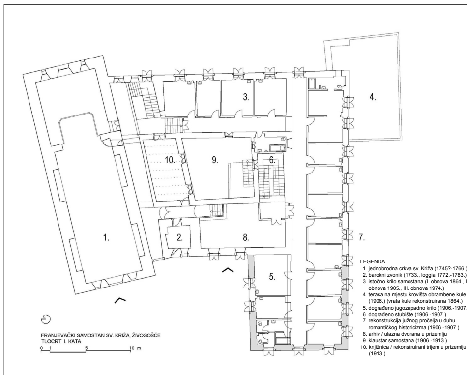
Sl.1. Tlocrt prvog kata samostanskog sklopa sv. Križa
