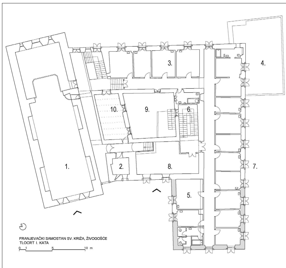
Sl. 2. Djelomični tlocrt prizemlja – postojeće stanje , list. 1. (B. Bezić, 1974.)
