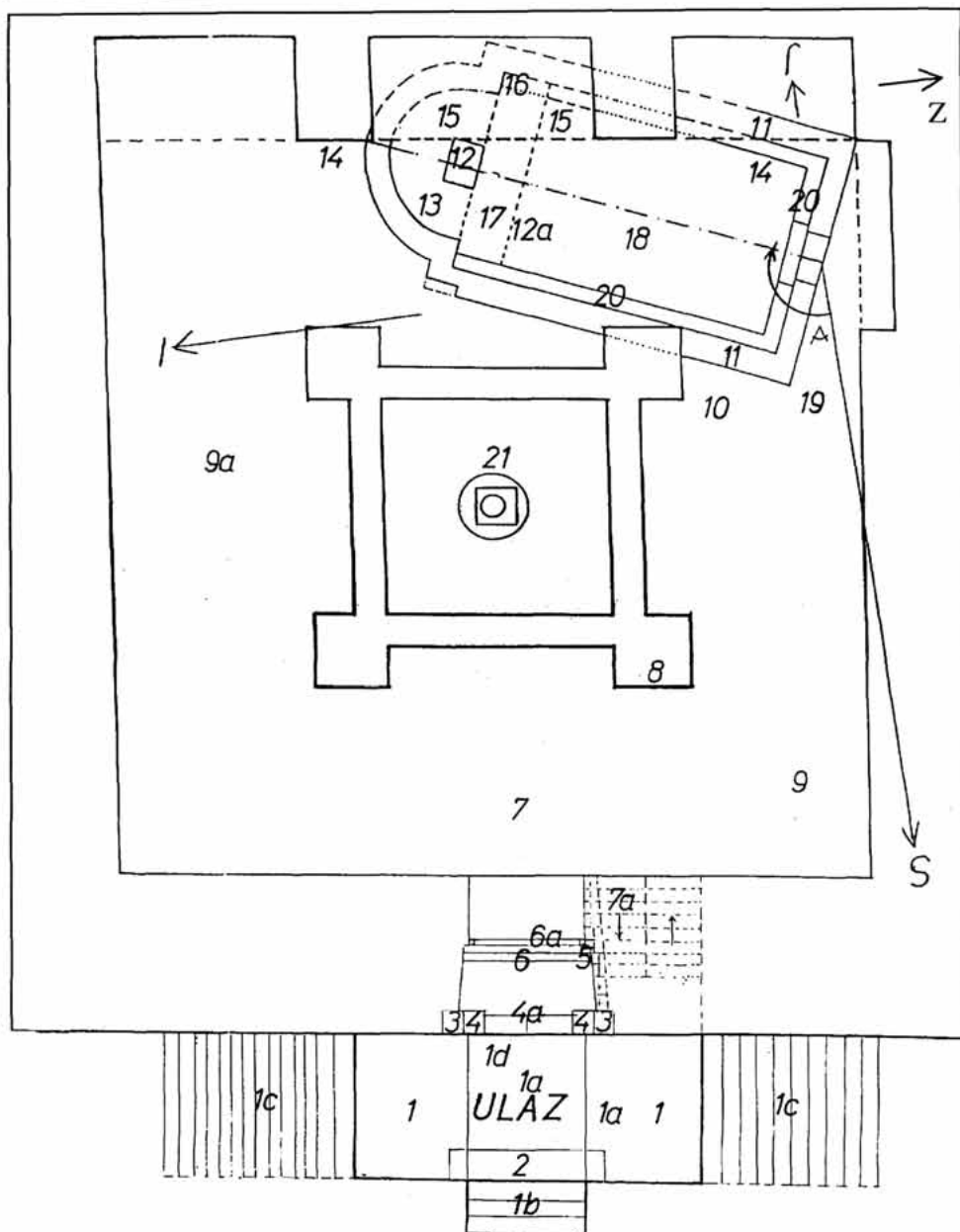
Sl. 1. Situacioni plan prizemlja tvrđave Nehaj s važnijim nalazima pronađenim pri restauraciji tvrđave. Izradili stručni suradnici: Ali Bakija, dipl. ing., Branka Rončević i Predrag Vukelić, geod. teh. Ureda za katastar u Senju, travanj 1999.
