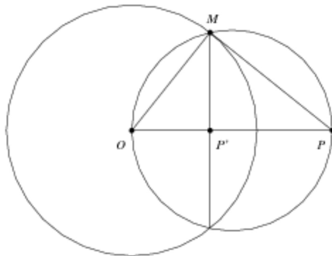
Slika 1: Inverzija je bijekcija i involucija.
