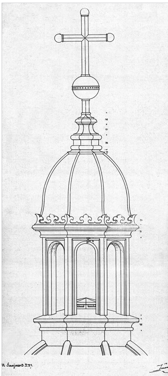
Josip Vancaš, Projekt za popravak lanterne na đakovačkoj katedrali.
