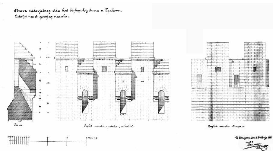
Josip Vancaš, Projekt za restauraciju srednjovjekovnog zida biskupskog sklopa u Đakovcu, 1888.
