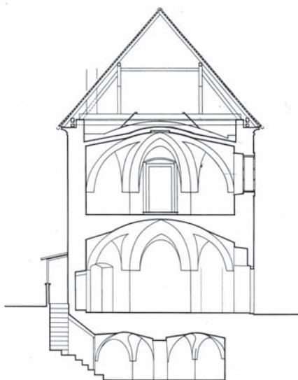
Slika 4. Poprečni presjek
