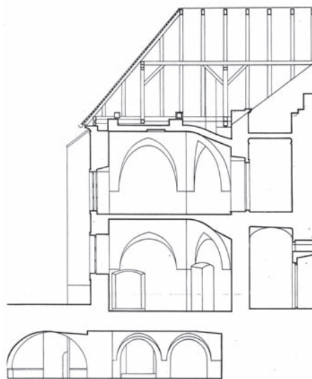
Slika 5. Uzdužni presjek
