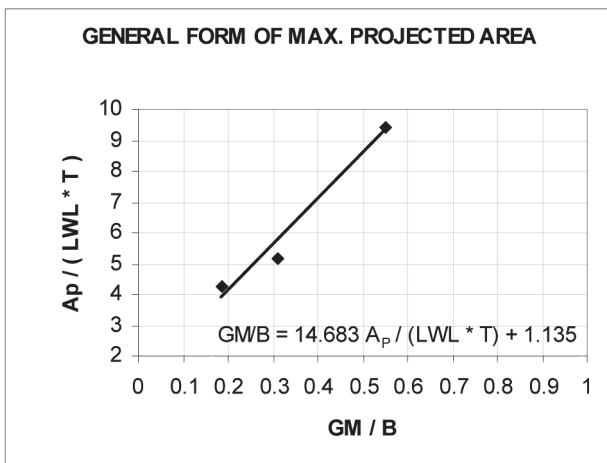
Figure 14 General form of the maximum projected lateral area Slika 14 Opći oblik najveće projicirane poprečne površine
