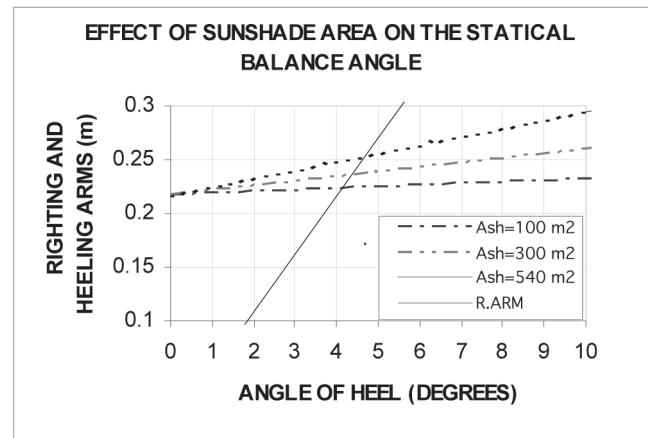
Figure 8 Effect of sunshade area on the static balance angle Slika 8 Učinak natkrivene površine na kut statičke ravnoteže
