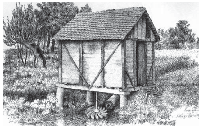
Sl. 3. Vodenica žličara na koju se voda dovodi preko cijevi te se mogu koristiti i najmanji vodotokovi (Matija Pokrivka, Mlinovi , n.dj., str. 46).
