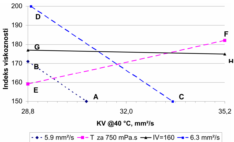
Slika 2: Područje formulacije za ISO VG 32 s VII 1
