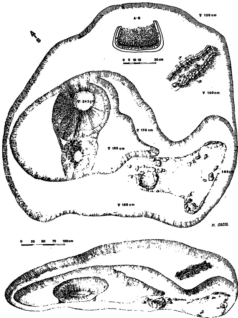
Sl. 5 : Zadubravlje, jama 12, keramičarske peći kao "cigara" i potkovičasta peć s kalotom-tlocrt, perspektiva i presjek
