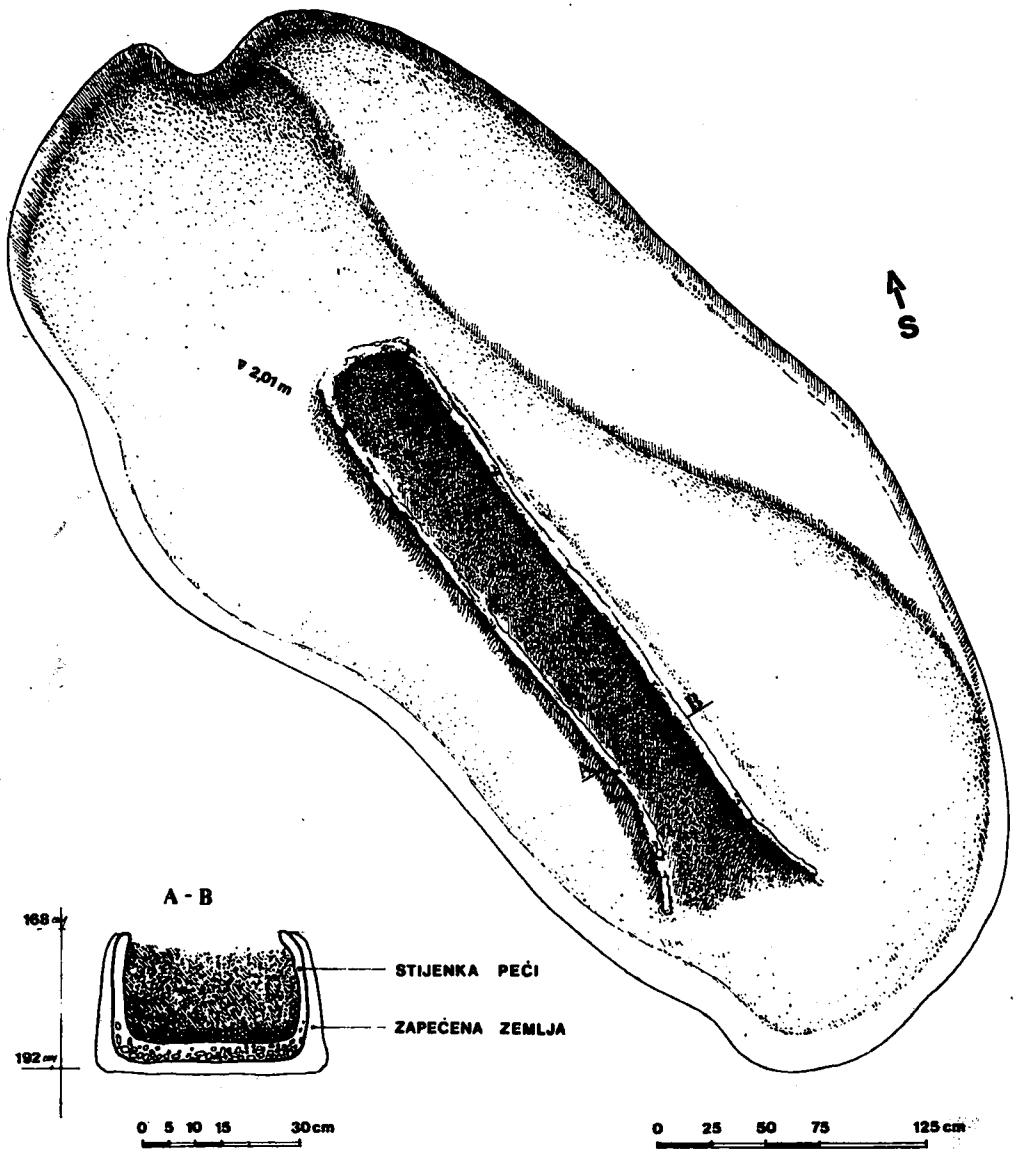
Sl. 6 : Zadubravlje, radni prostor 14 i keramičarska peć kao "cigara" -tlocrt i presjek Abb 6: Zadubravlje, Arbeitsfläche 14 und Keramikofen in Form einer "Zigarre" – Grundriß und Querschnitt
