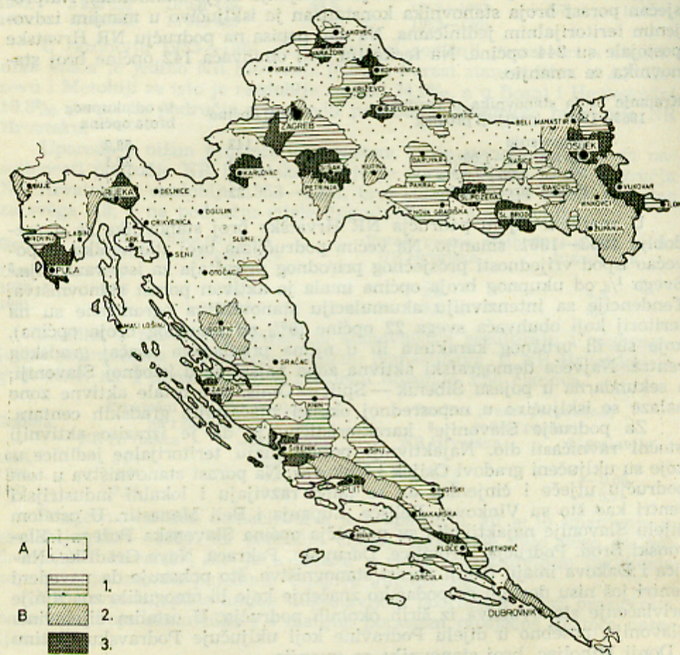
Sl. 1. Kretanje broja stanovnika na području NR Hrvatske u razdoblju 1953.—1961. A — područja u kojima se broj stanovnika smanjivao; B — područja u kojima se broj stanovnika povećavao uz godišnji prosjek porasta: 1) 0.1 — 1.05% 2) 1.06 — 2.00% i 3) 2.1% i više.
