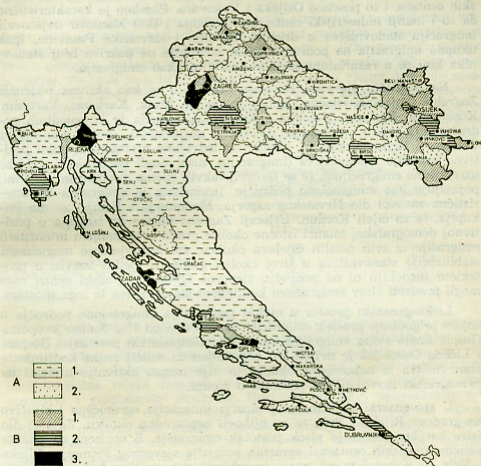
Sl. 2. Migracije stanovništva na području NR Hrvatske u razdoblju 1953.—1961. A — emigracija (godišnji prosjek): 1. preko 1.1‰ i 2. do 1‰; B — Imigracija (godišnji prosjek): 1. do 1‰, 2. 1.1 do 2.0‰ 3. preko 2.0‰.
