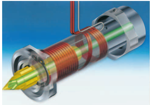
SLIKA 3. Hascova topla mlaznica Rapid Shot Z 3500/...
