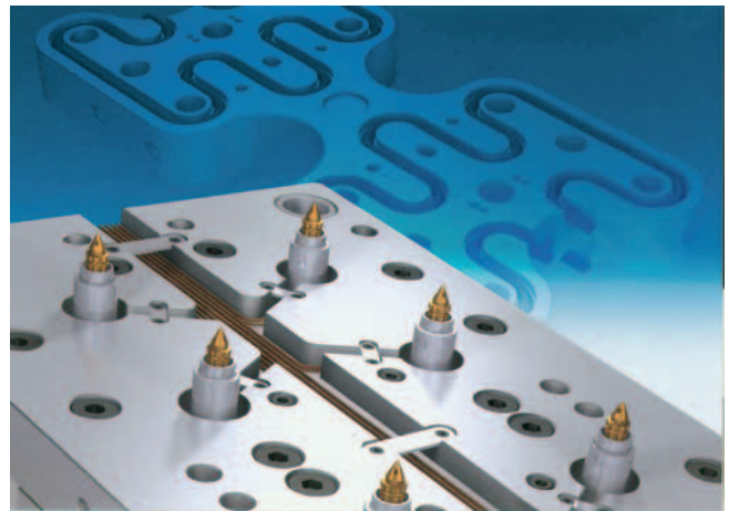
SLIKA 5. Hascov topli dio kalupa
