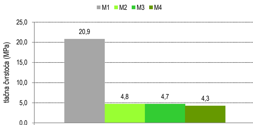
Slika 11 - Tlačne čvrstoće morta nakon 2 dana starosti uzoraka
