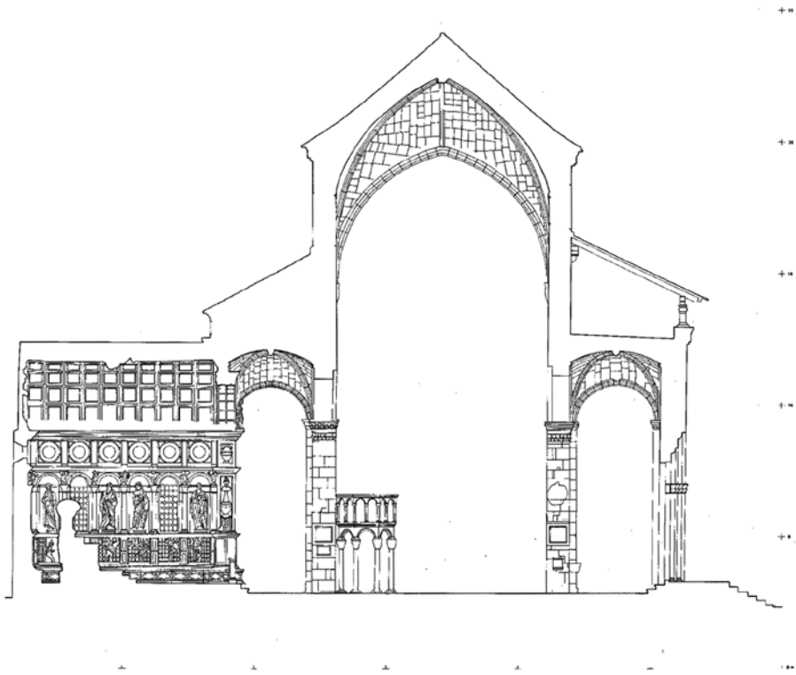
Poprečni presjek kroz trogirsku katedralu (Zavod za fotogrametriju Geodetskog fakulteta u Zagrebu)
